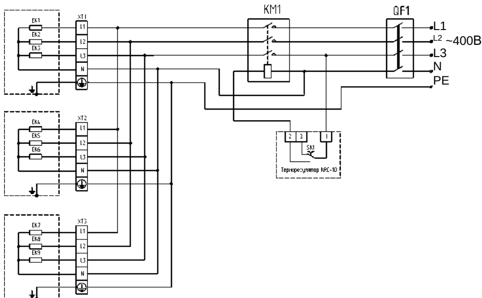
Рис. 2 Обогреватель для TIR-T3.0-54, TIR-T4.5-54, TIR-T6.0-54
