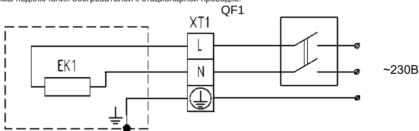
Рис. 1 Обогреватель для TIR-T1.0-54, TIR- T1.5-54, TIR- T2.0-54
