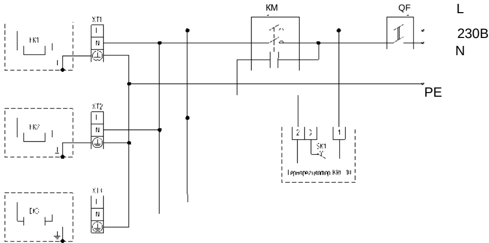
Рис. 1 Обогреватель для TIR-T1.0-54, TIR-T1.5-54, TIR-T2.0-54
