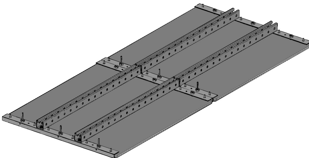
Рисунок 5 - Монтаж шести обогревателей IRS-G083-54 с кронштейном МК-6
